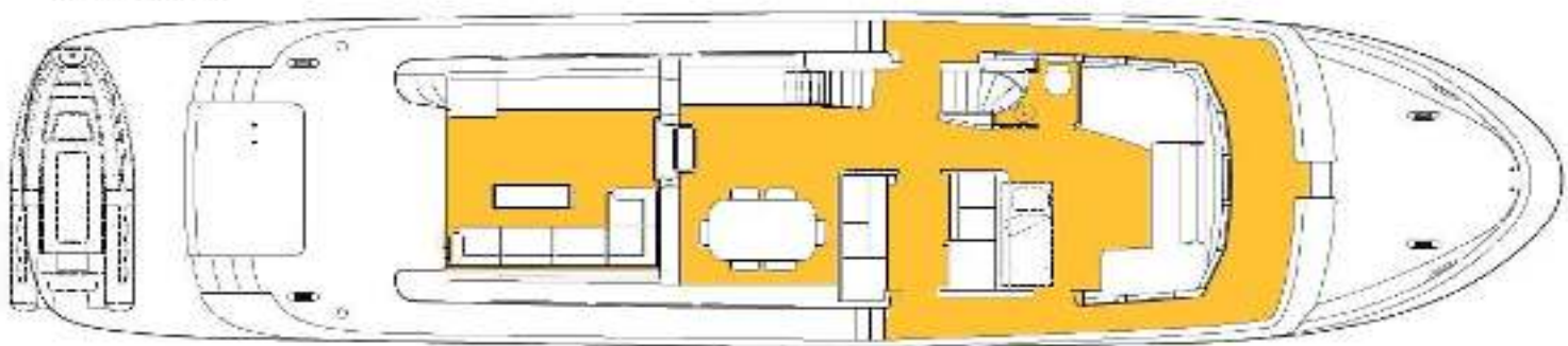
PONTE DI COPERTURA
