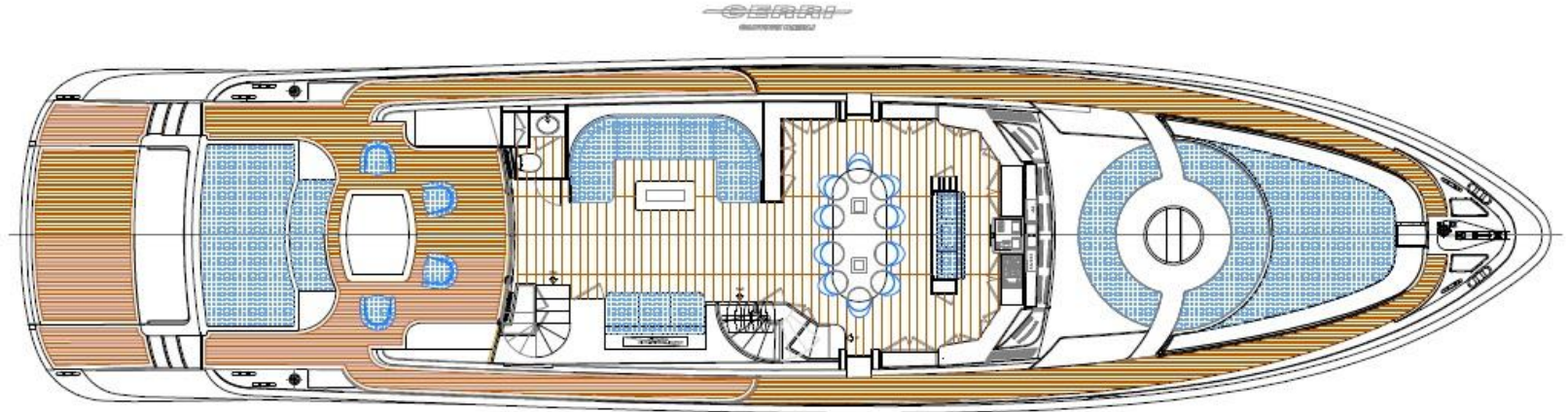
PONTE COPERTA
