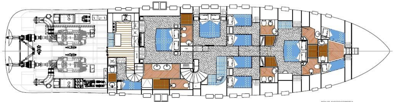
PONTE SOTTOCOPERTA
